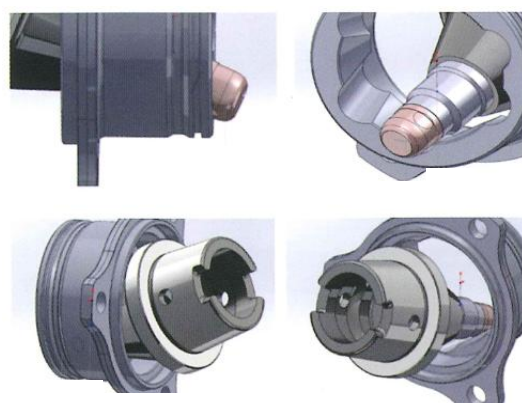
アウターレース
